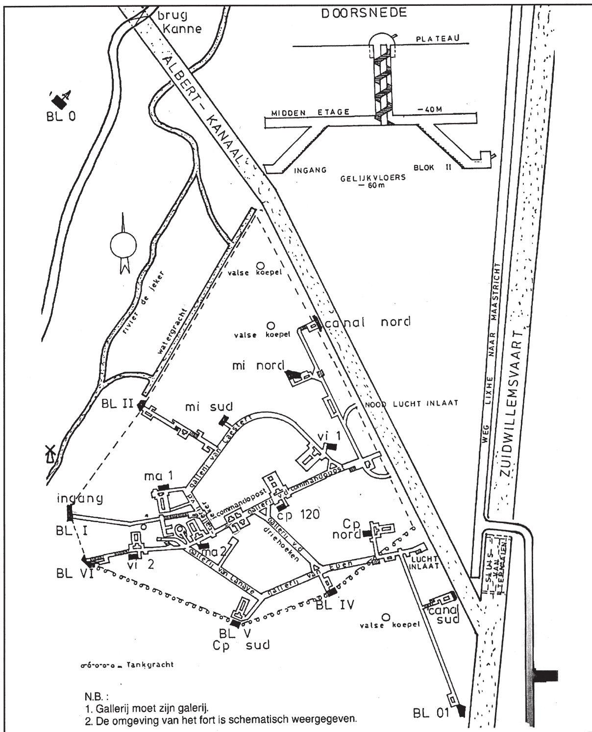
Plattegrond Fort Eben-Emael
