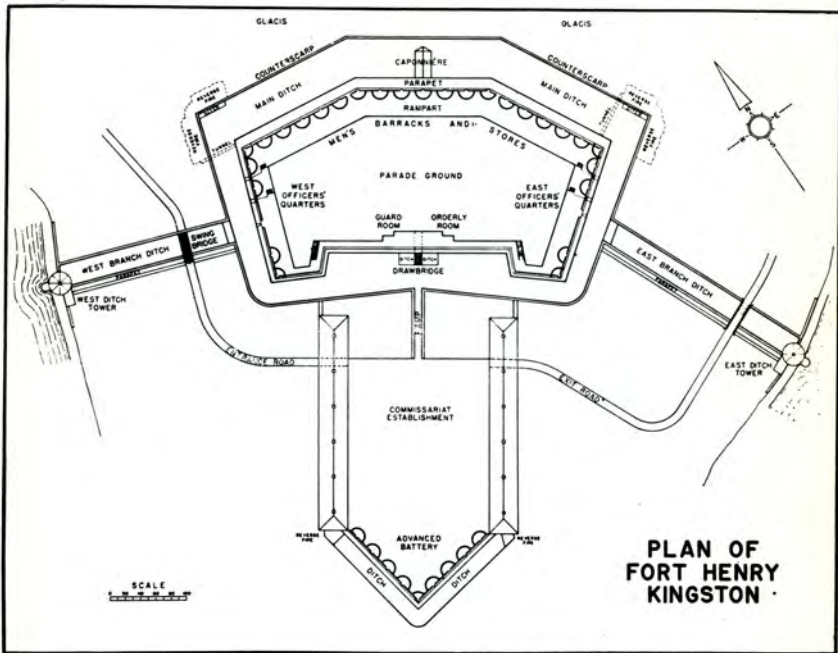
(a) Plan Old Fort Henry bij Kingston (1832-'36)
